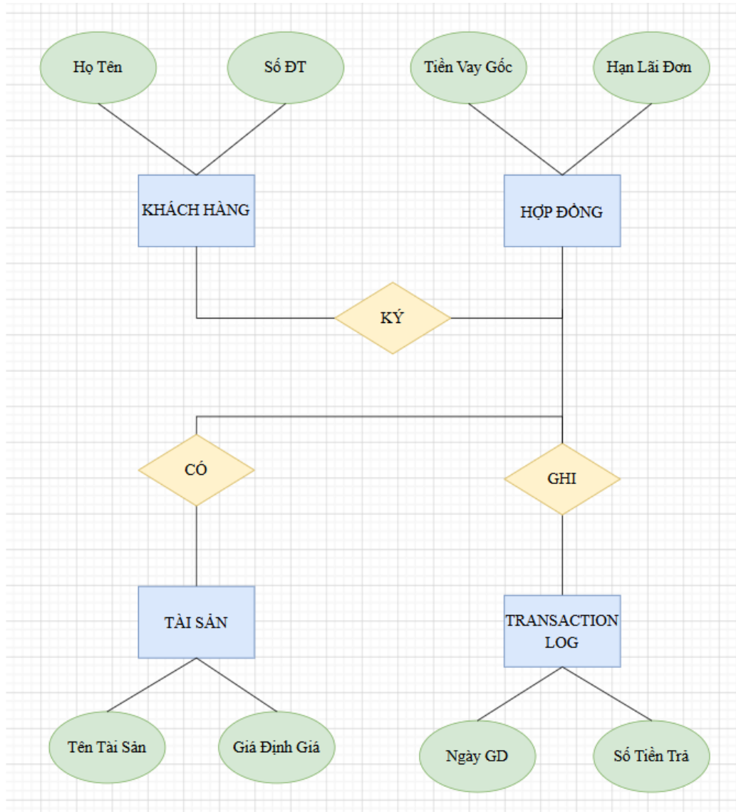
Sơ đồ ERD của quản lý cầm đồ
